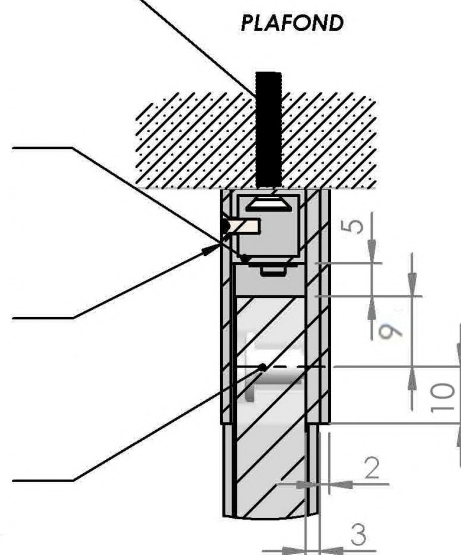
DÉTAIL B ECHELLE 1 : 2
