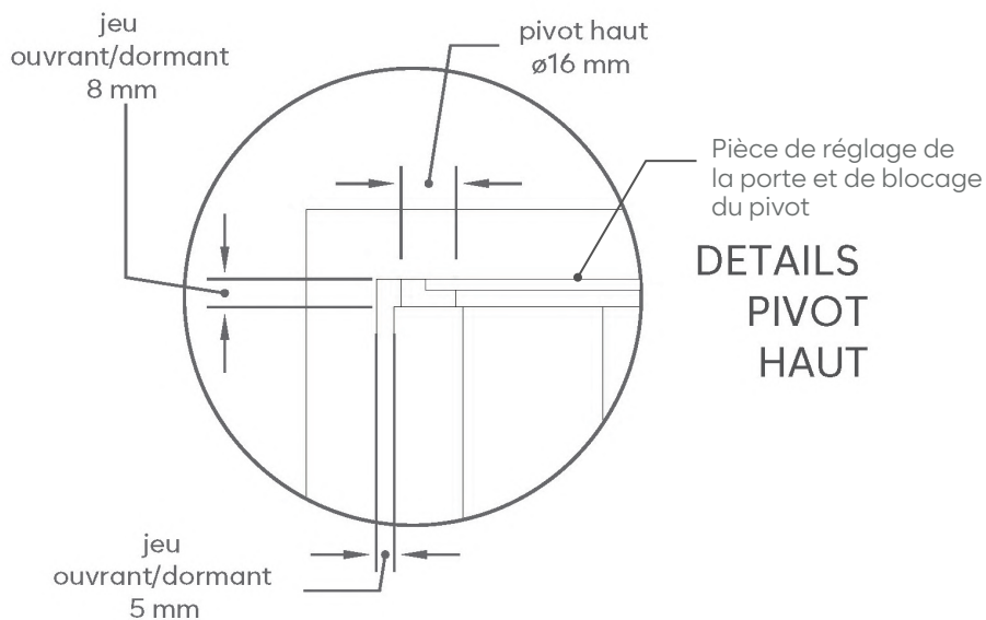
Pièce de réglage de la porte et de blocage du pivot 100 x 20 ép. 3 mm
