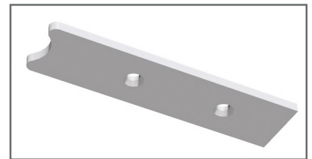
Pièce de réglage de la porte et de blocage du pivot 100 x 20 ép. 3 mm
